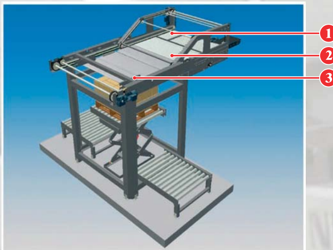
Un paletizador NEDPACK Highrunner estándar
